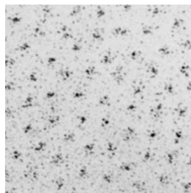
VORTEX GLASS
