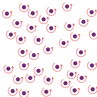
VORTEX GLASS
